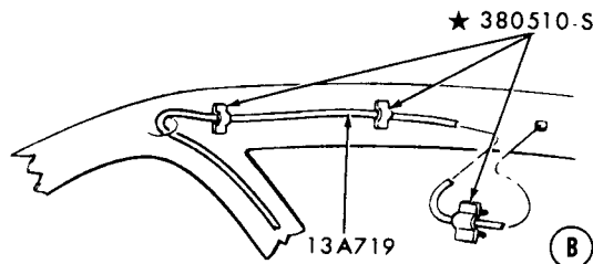
DOME LAMP 1971/72 PINTO
